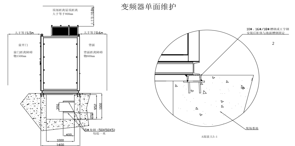
变频器单面维护 电缆沟槽及地上沟槽断面图
