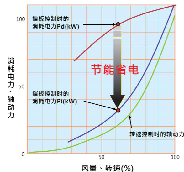
■ 耗电特性曲线
