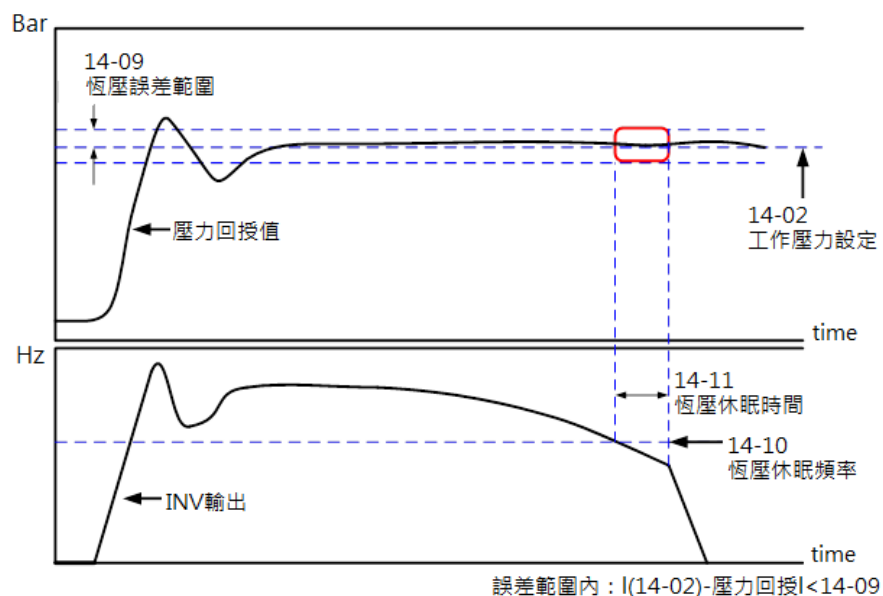
恆壓停機示意圖
