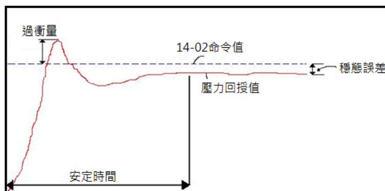
壓力回授值示意圖
