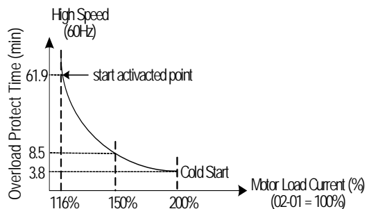
馬達過載保護曲線(標準馬達範例)
