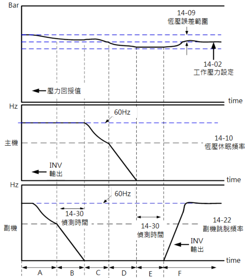
休眠停止交換主副機動作流程
