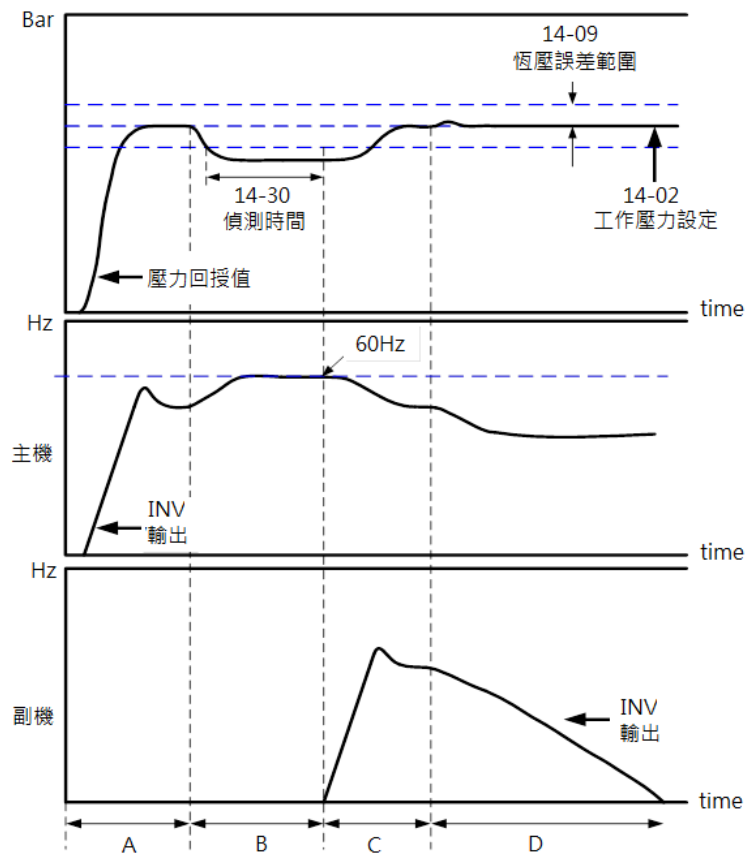
雙泵浦啟動功能流程
