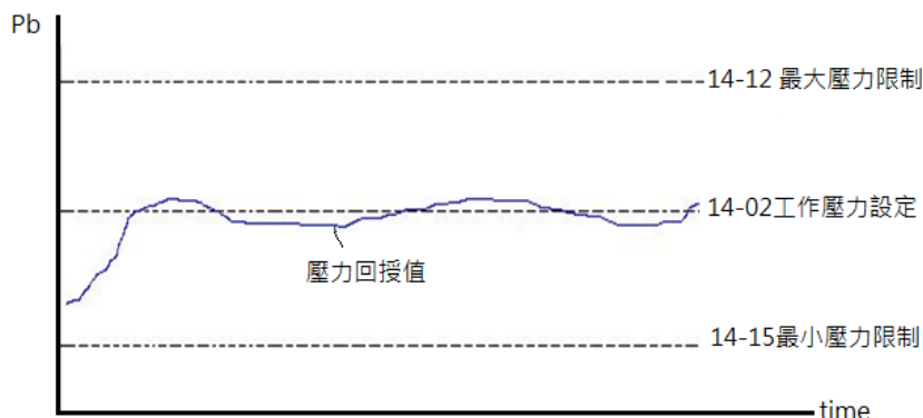
壓力回授限制示意圖
