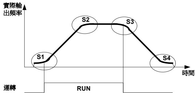
有 S 曲線的加減速特性
