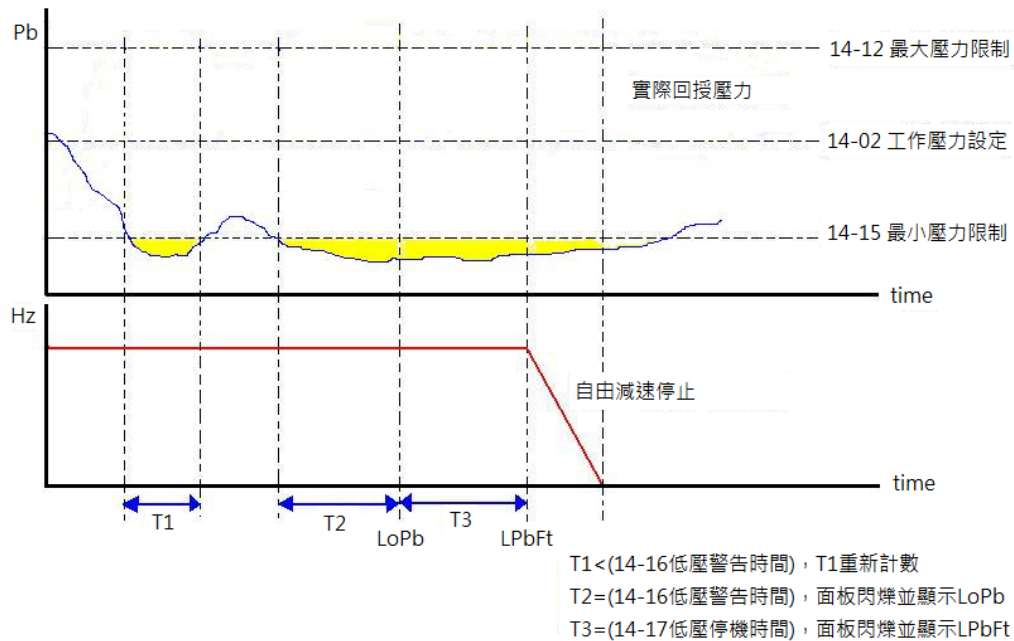
低壓限制警告停機示意圖
