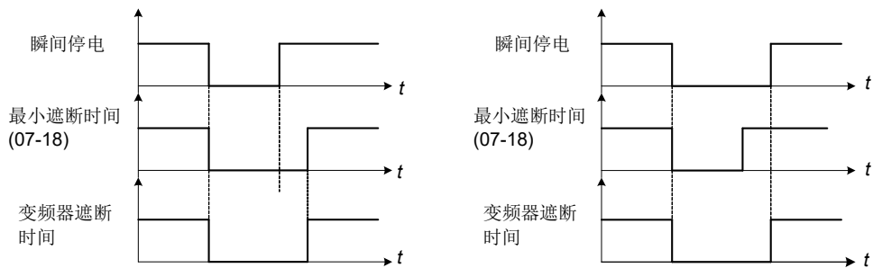
(a) 当最小遮断时间（07-18）大于瞬间停电时间 (b) 当最小遮断时间（07-18）小于瞬间停电时间
