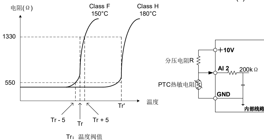
(b) PTC热敏电阻连接示意图
