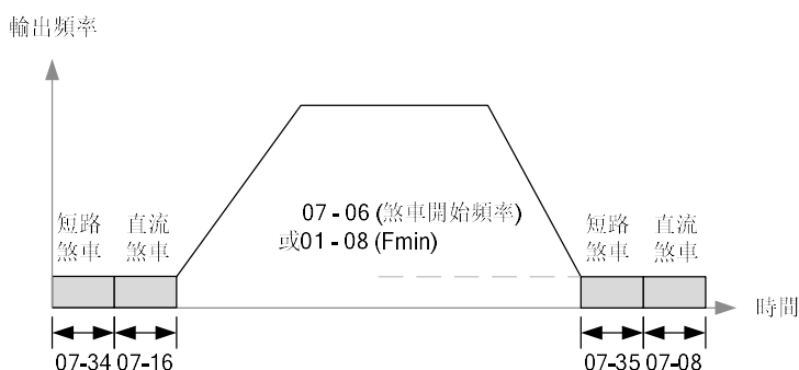
图4.3.57b PMSLV的煞车动作
