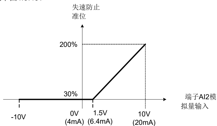
图4.3.43 运转期间失速防止准位调整
