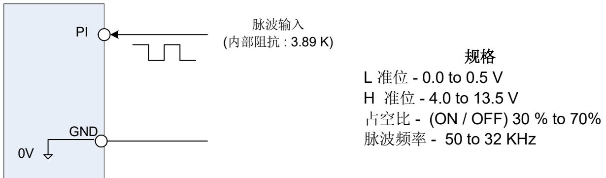
图 4.3.5 脉波输入之频率参考功能
