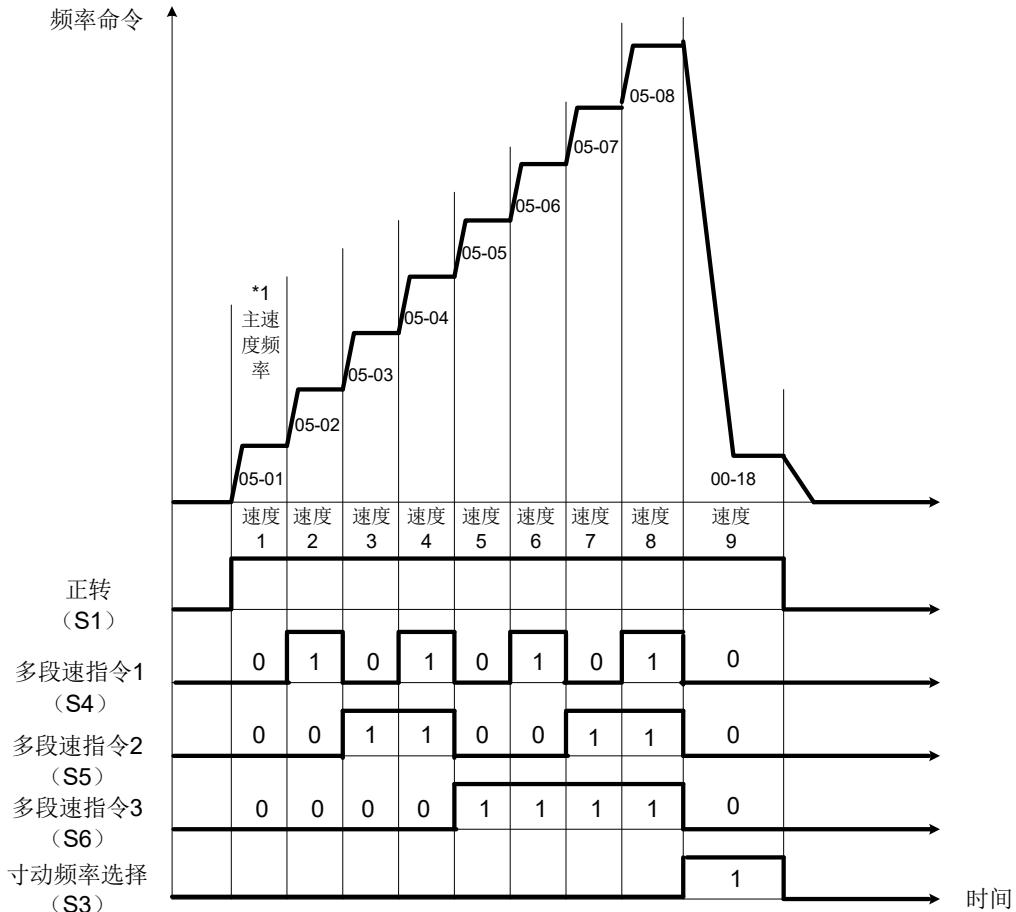
9段速时序图
