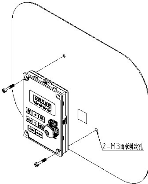
LED 数字操作器之安装方式 1 尺寸图
