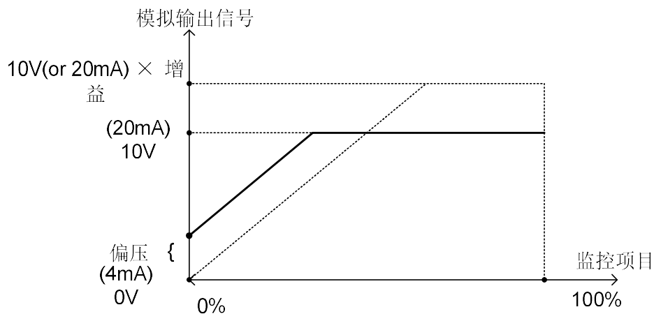
图4.3.48 模拟输出准位调整
