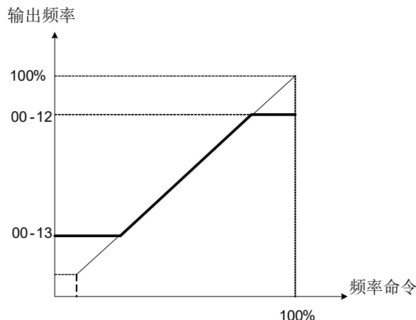
图 4.3.6 参考频率上下限
