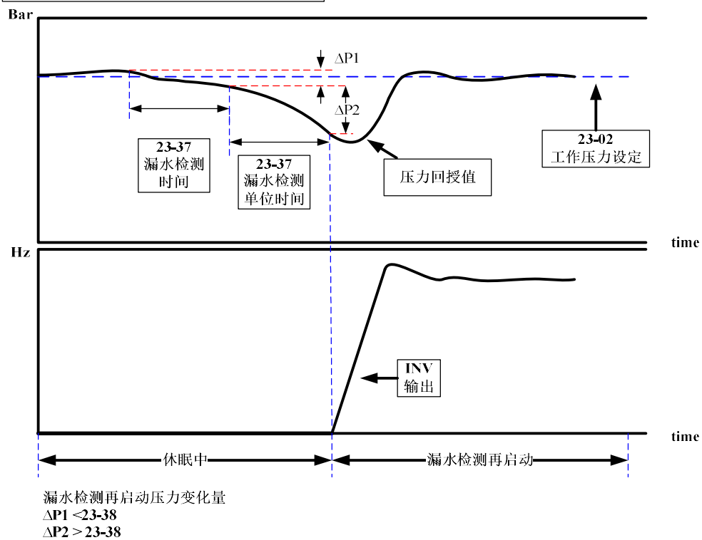
漏水检测 Case1: 压力变化量大于23-38
