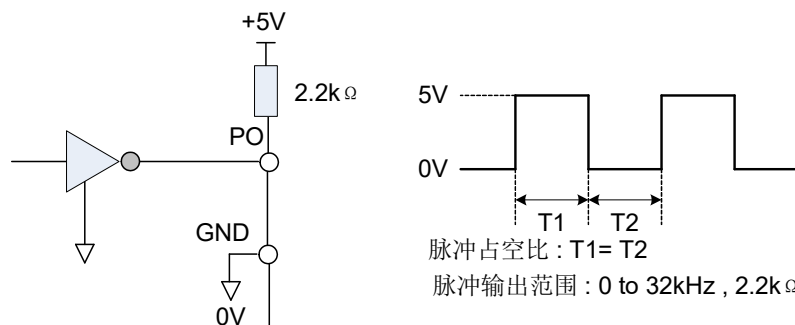
图 4.3.28 脉波输出信号准位
