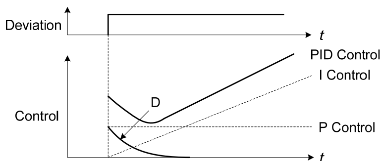
圖 4.3.78 PID 控制操作
