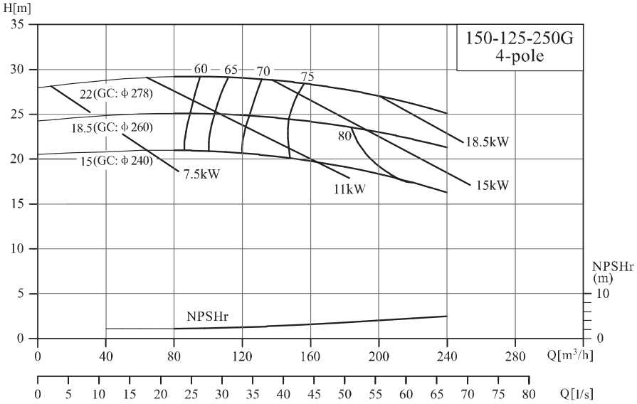
NIS/NISF150-125-250G/150-125-315(Q)
