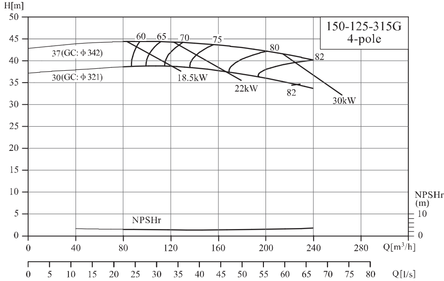
NIS/NISF150-125-315G/150-125-400(Q)
