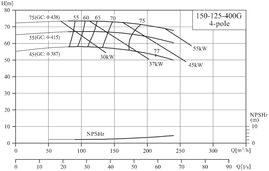
NIS/NISF150-125-400G/200-150-250(Q)
