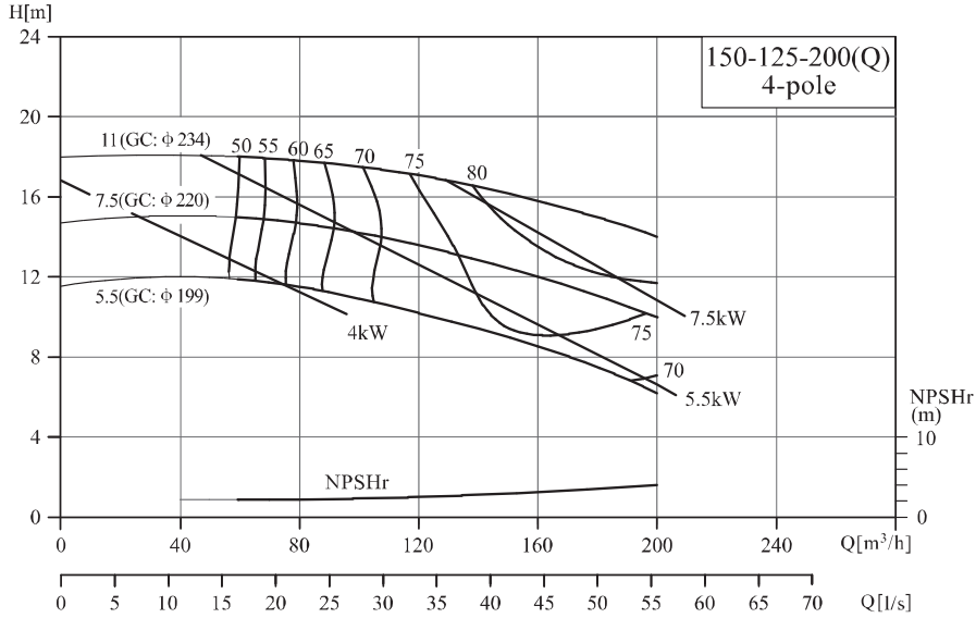
NIS/NISF150-125-200(Q)/150-125-200G
