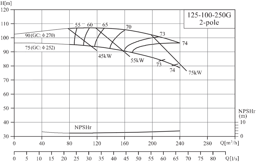
NIS/NISF125-100-250G/125-100-315G
