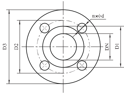
NIS/NISF*G,NIS/NISF*(Q) Flange
