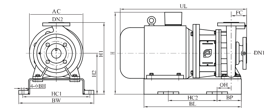
NIS/NISF*G,NIS/NISF*(Q) Dimension table
