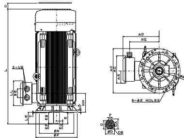
外形及安装尺寸图
