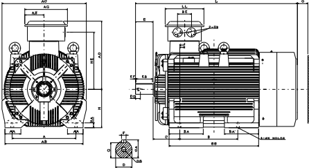
外形及安装尺寸图
