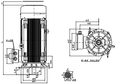
外形及安装尺寸图
