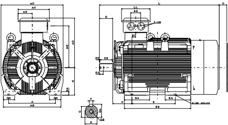
外形及安装尺寸图
