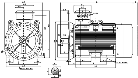
外形及安装尺寸图
