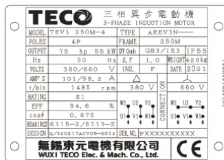
中英文铭板
