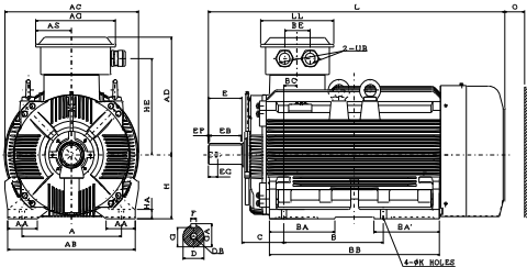
外形及安装尺寸图
